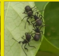
Hausa – yayan bakin karbobo Français – Larves punaise noire Scientifique – Anoplocnemis curvipes
