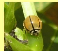
Français – Coccinelle Hausa -Mai shayi ukku rawaya Scientifique – Cheilomenes vicina
